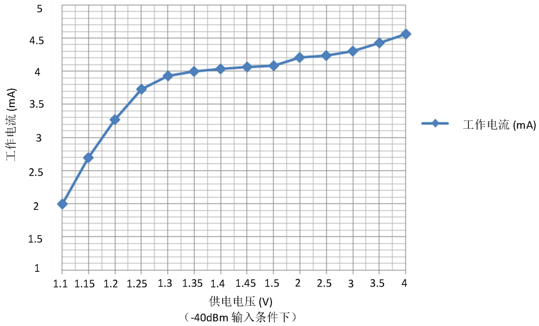
图 3. 工作电流与供电电压的关系曲线
