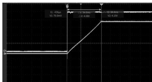
MSR040: 10µF 负载电容时的启动时间
