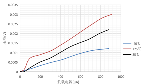
MSR040: 不同温度条件下, 压降与负载电流间的关系
