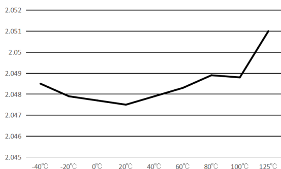
MSR020: 输出电压温漂曲线 (VCC=5V)
