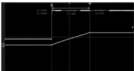
MSR020: 10µF 负载电容时的启动时间
