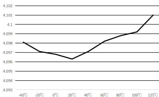
MSR040: 输出电压温漂曲线 (VCC=5V)
