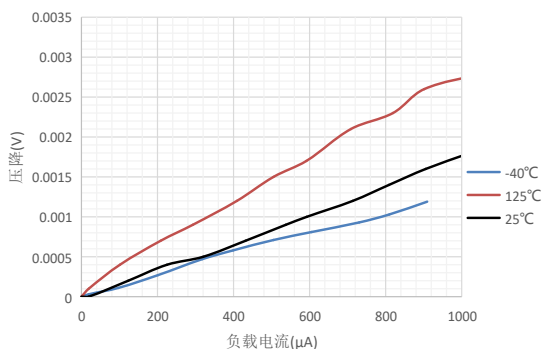
MSR020: 不同温度条件下, 压降与负载电流间的关系
