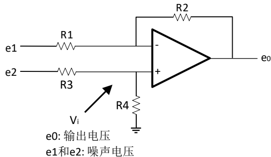
噪声抑制原理
