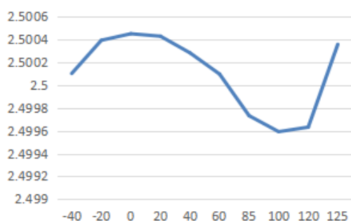
MSR025: 输出电压温漂曲线 (VCC=5V)
