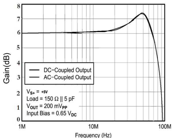
图 1. 频率响应
