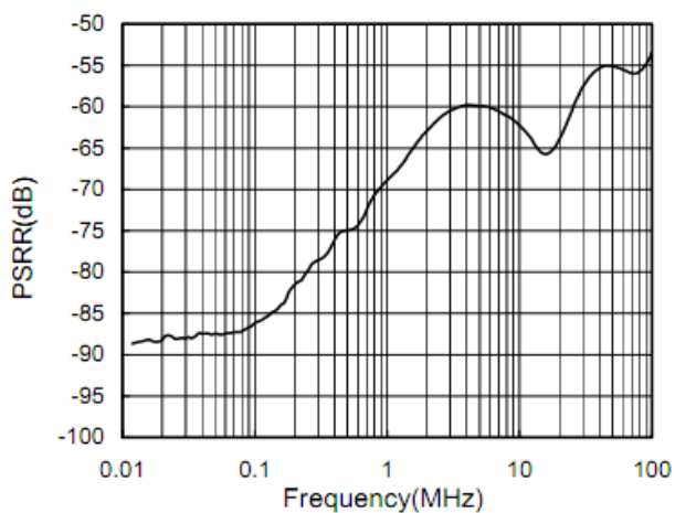
图 5. 电源电压抑制比与频率的关系 (有旁路电容)
