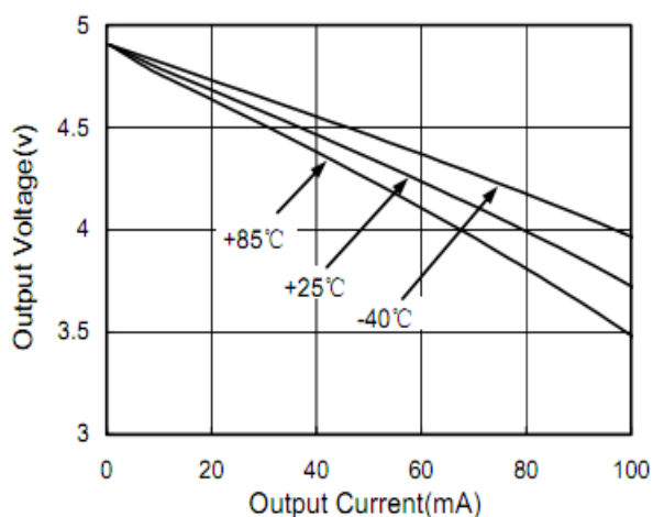
图 11. 正隔离输出电压幅度与输出电流的关系
