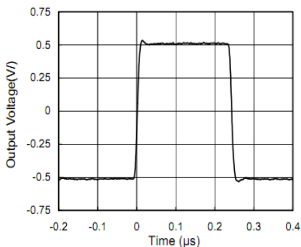
图 3. 大信号阶跃响应
