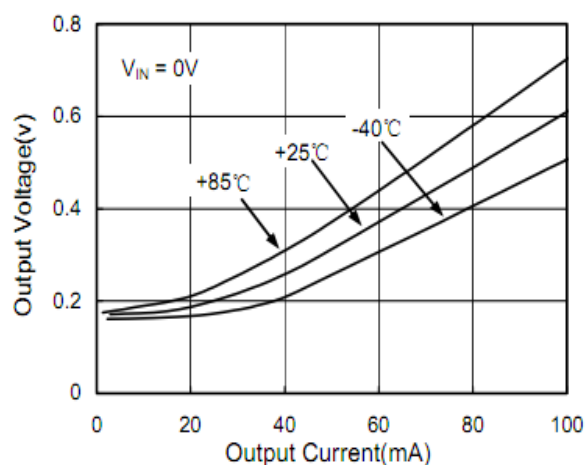
图 12. 负隔离输出电压幅度与输出电流的关系
