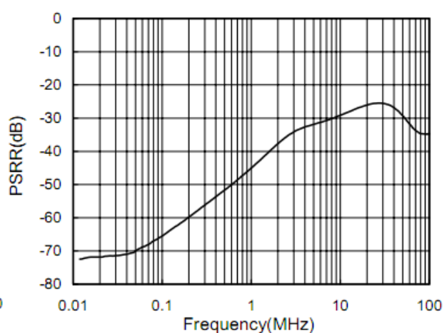
图 6. 电源电压抑制比与频率的关系 (无旁路电容)
