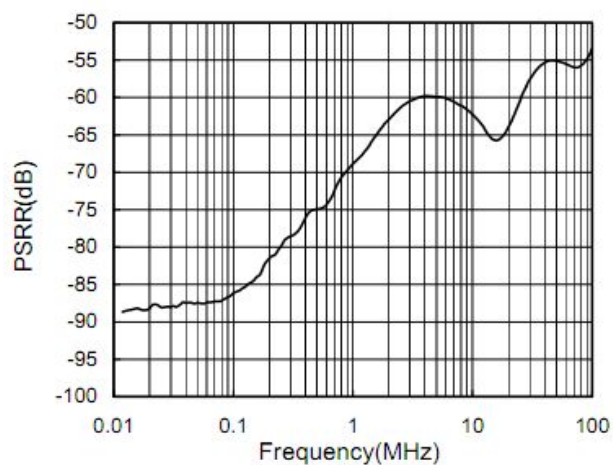
图 6. 电源抑制比与频率的关系 (有旁路电容)
