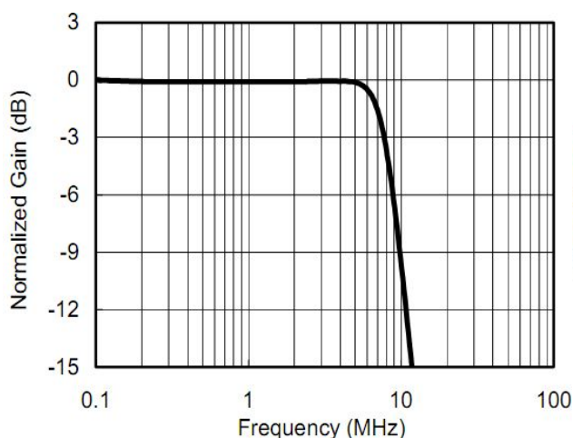
图 2. 频率响应
