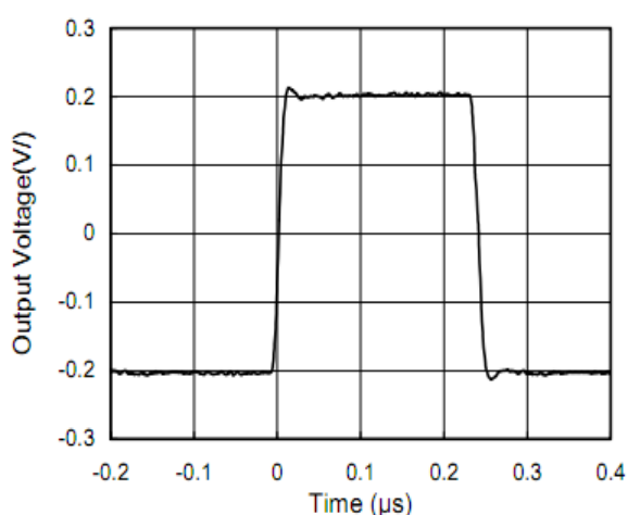
图 4. 小信号阶跃响应
