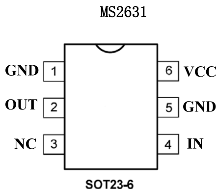
SOT23-6 封装图
