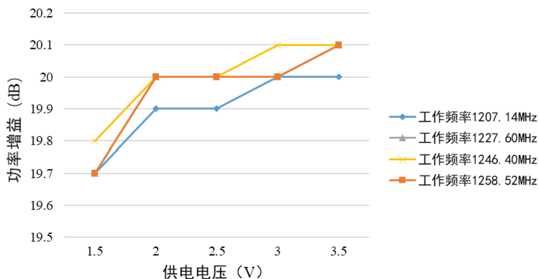
图二、功率增益与供电电压的关系曲线
