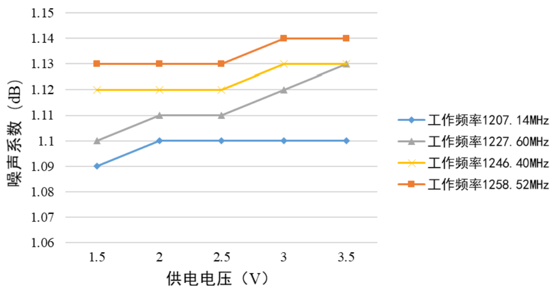
图一、噪声系数与供电电压的关系曲线
