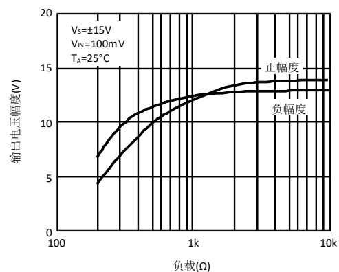
图 8. 输出电压摆幅 VS. 负载
