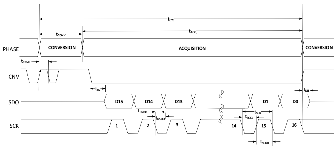
接口时序图
