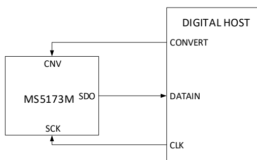
接线图
