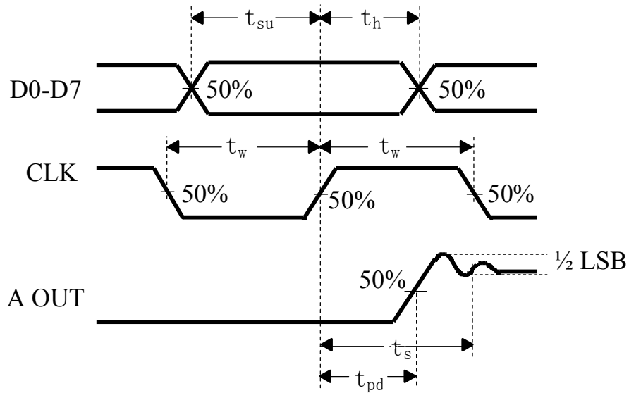
图1 电压波形
