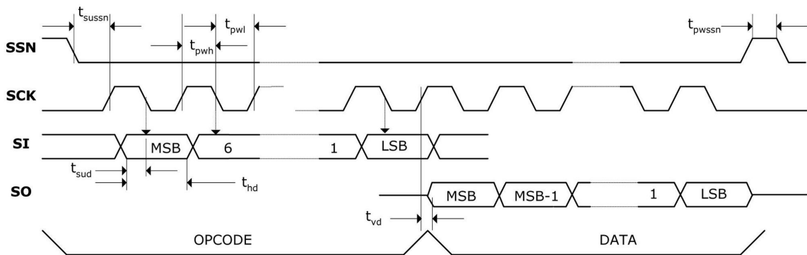
图 2.SPI 读时序
