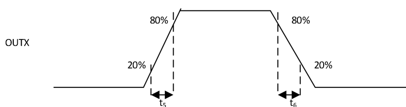
图 2. MS3111D 输入输出时间参数 2
