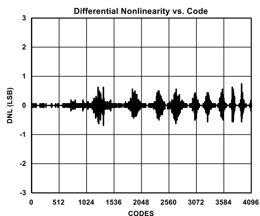
图 3. 微分非线性与码的关系, DR=01
