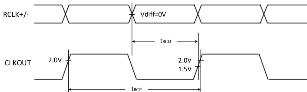
图 8. 输入时钟与输出时钟间延迟
