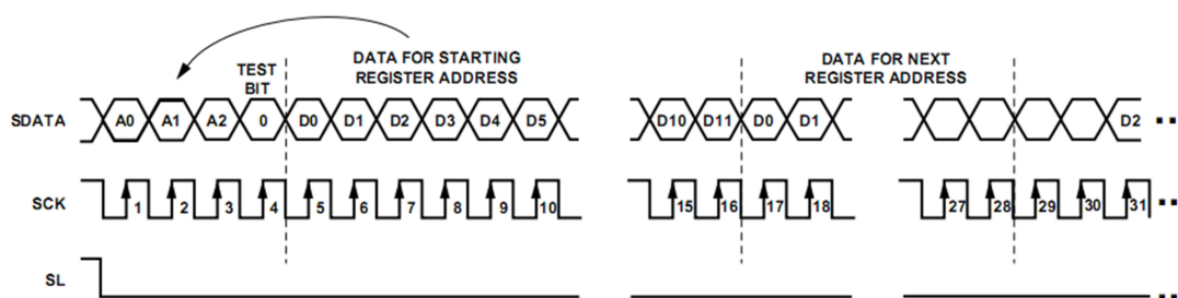
串口连续写操作
