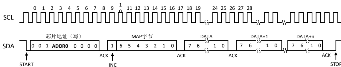
图 1. 控制端口时序，I 2 C 从模式写
