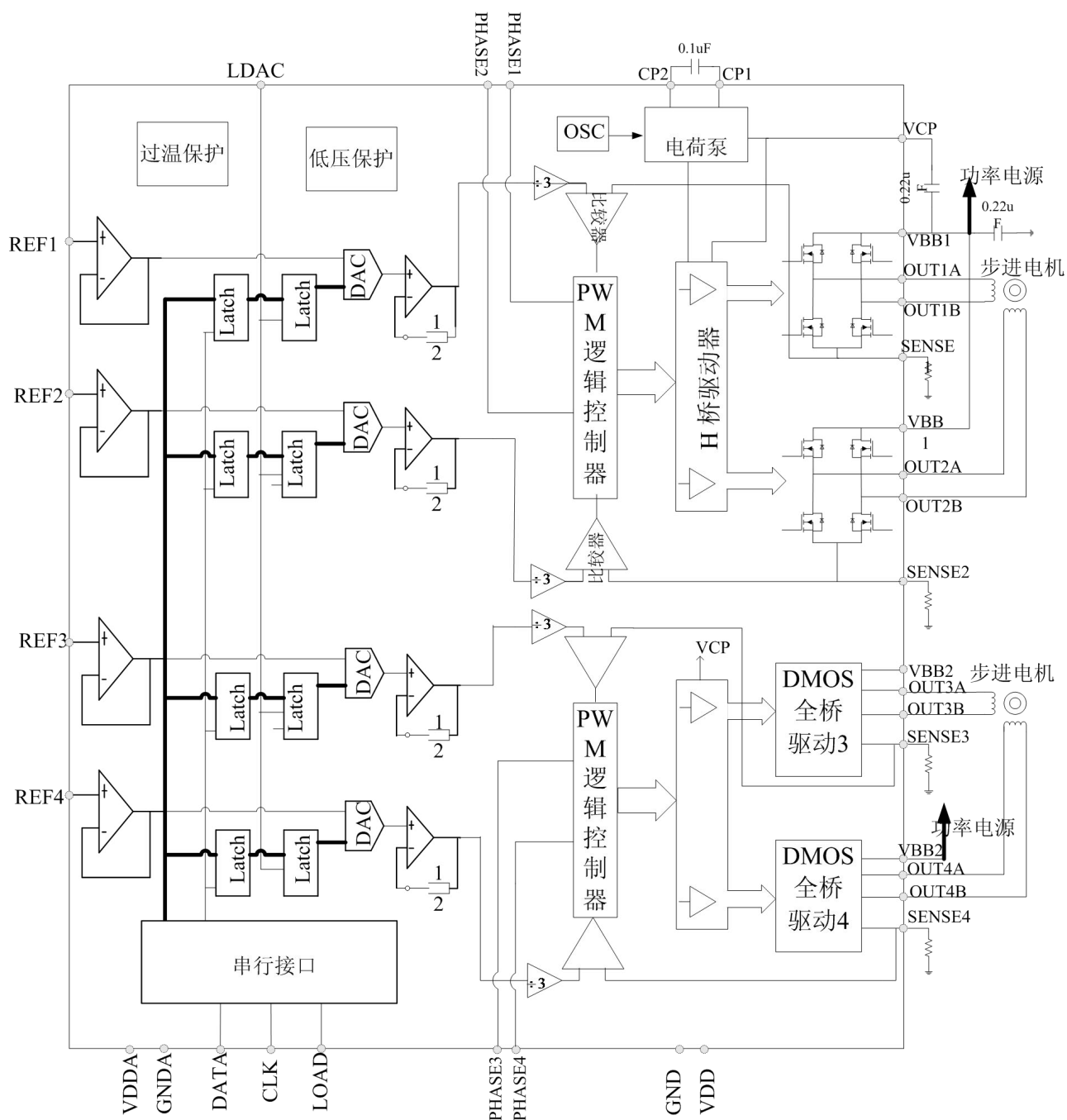
图 1 内部框图
