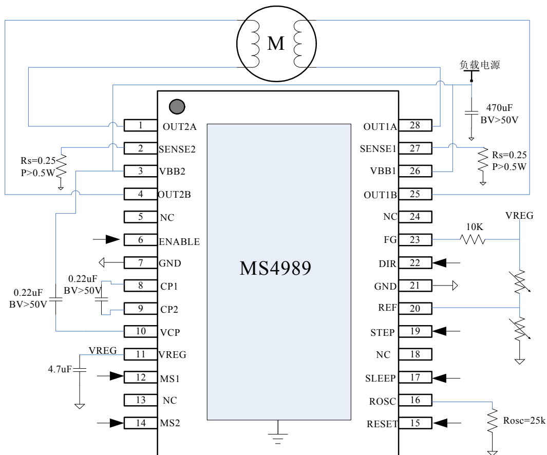
典型应用电路图
