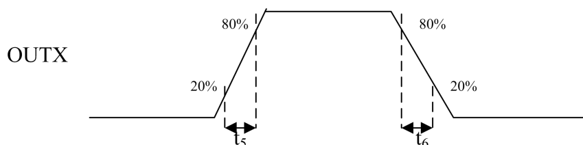
图 3 MS3010 输入输出时间参数 2
