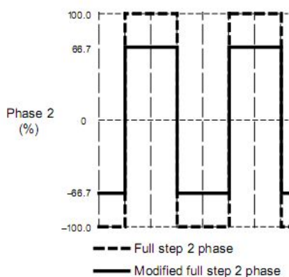
图4 全步进循序
