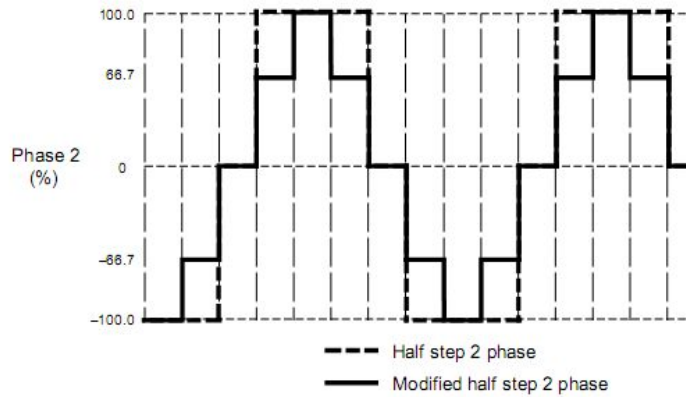
图5 半步进循序
