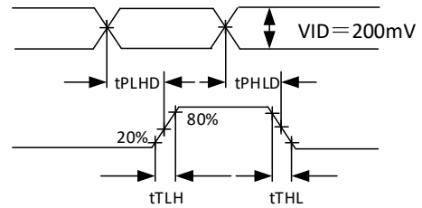
图 2. 传输延时和转变时间波形图
