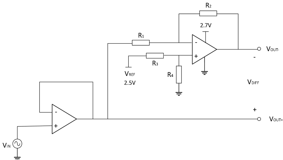
图 1. 单端输入到差分输出的转换电路
