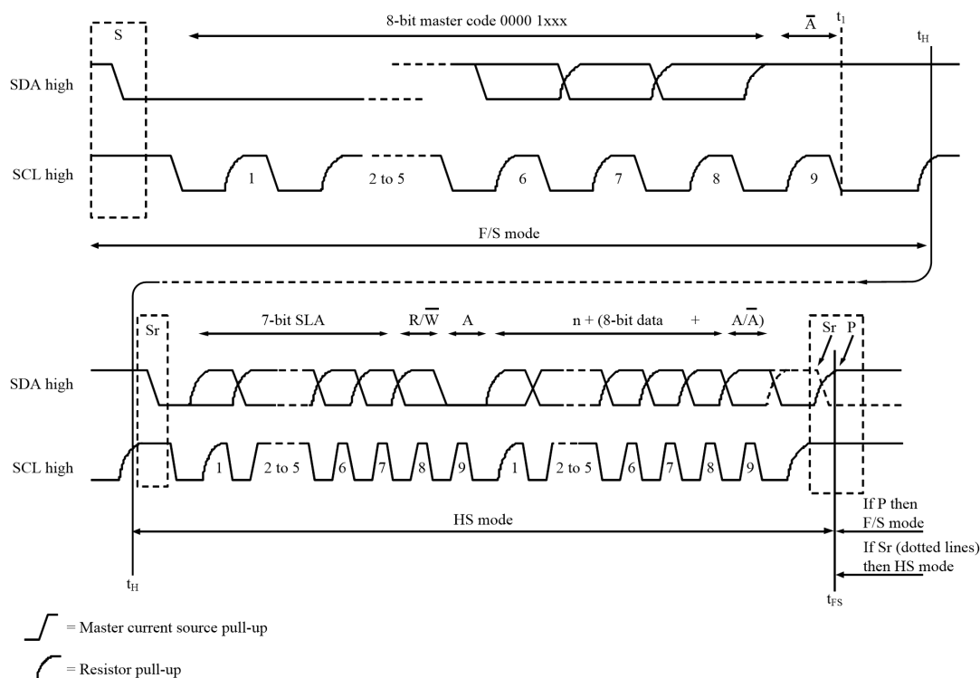
图 19. I 2 C 总线高速模式协议帧
