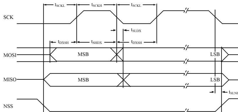
图 2. SPI 时序图
