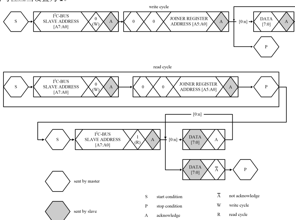
图 17.寄存器读和写访问
