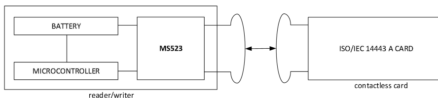
图 4. MS523 读写模式
