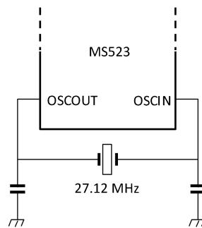
图 22. 石英晶体的连接
