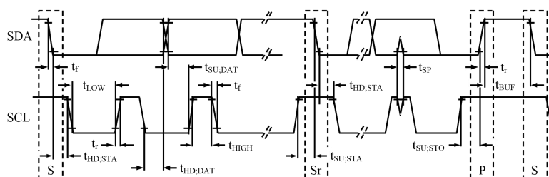
图 3. I 2 C 总线上快速和标准模式器件的时序
