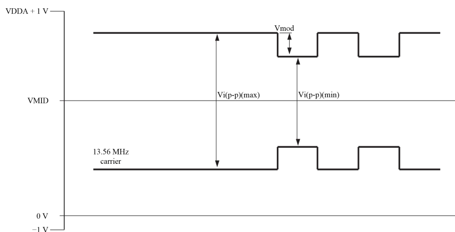
图 1. 管脚 RX 输入电压范围
