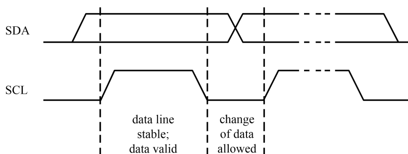
图 12. I 2 C 总线的位传输
