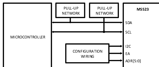
图 11. I 2 C 总线接口
