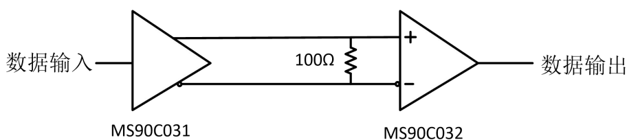
图 5. 典型应用图
