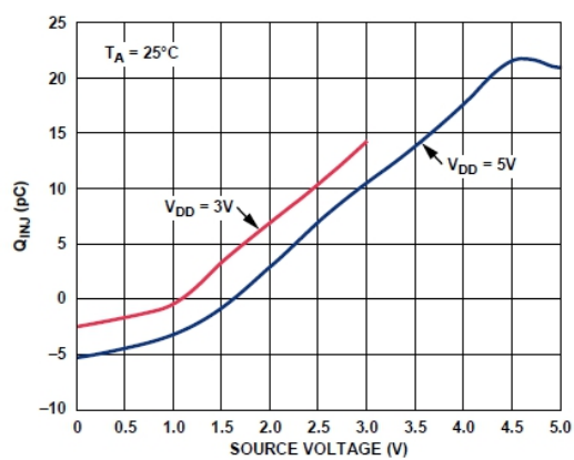
电荷注入 VS. S 端电压曲线
