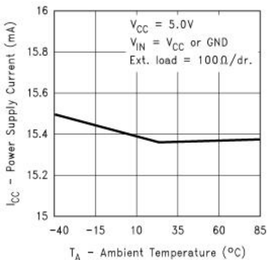
电源电流 vs. 温度（100Ω负载）
