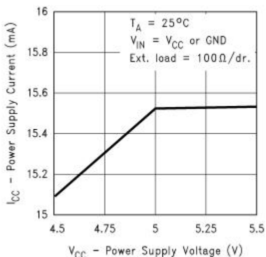
电源电流 vs. 电源电压（100Ω负载）
