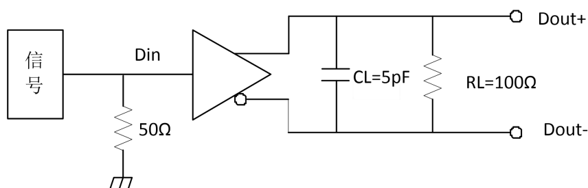
图 2. 传输延时和沿转变时间测试电路
