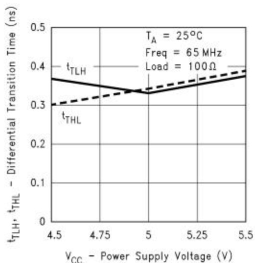
差分传输沿时间 VS. 电源电压
