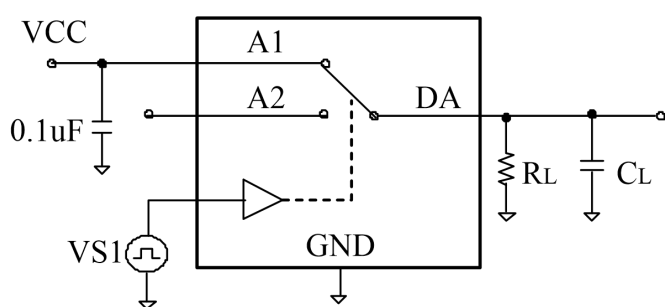
测试电路 3. 先断后通时间( t_D )
